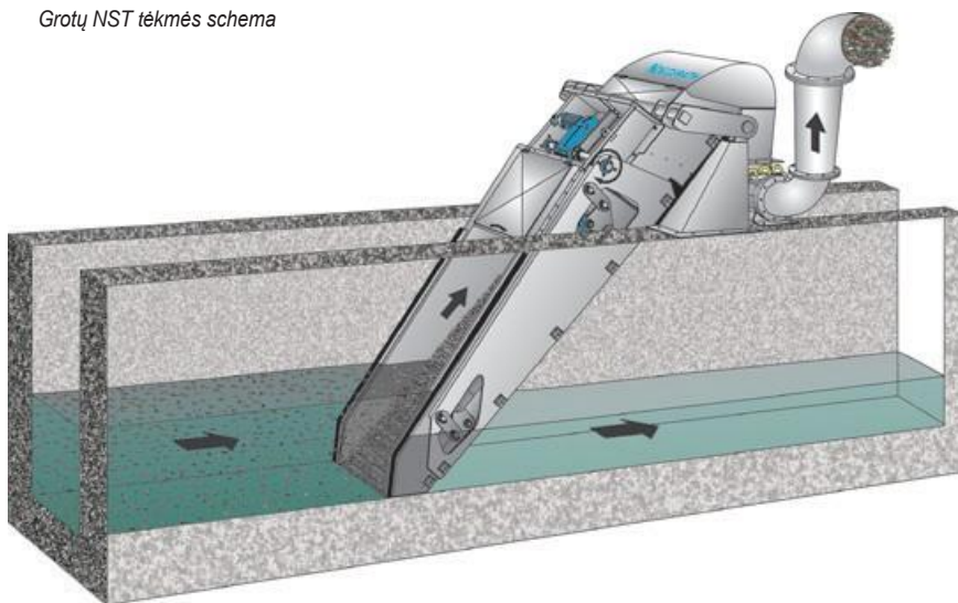
Grotų NST tėkmės schema
